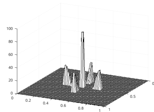
(d) Lagrange multiplier \bar{\lambda}
